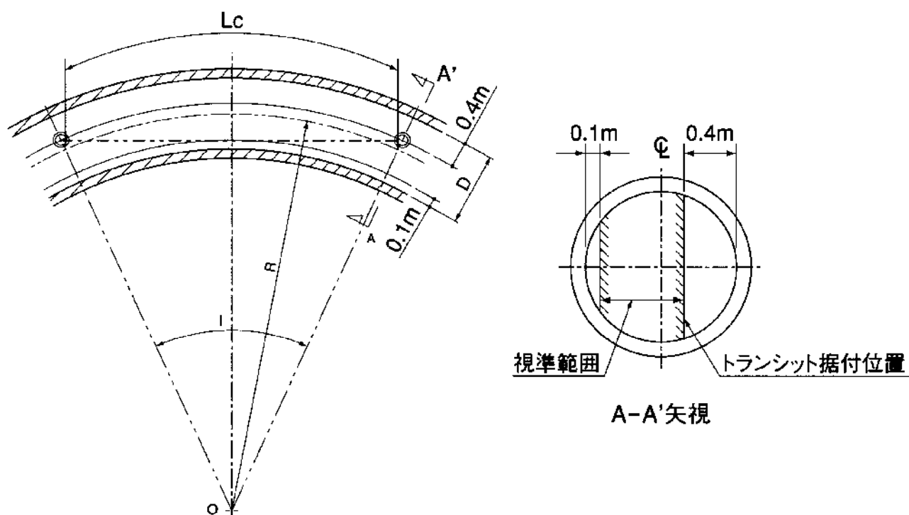
図 1－1 曲線区間での 1 回当たりの測量長・曲線長の関係
