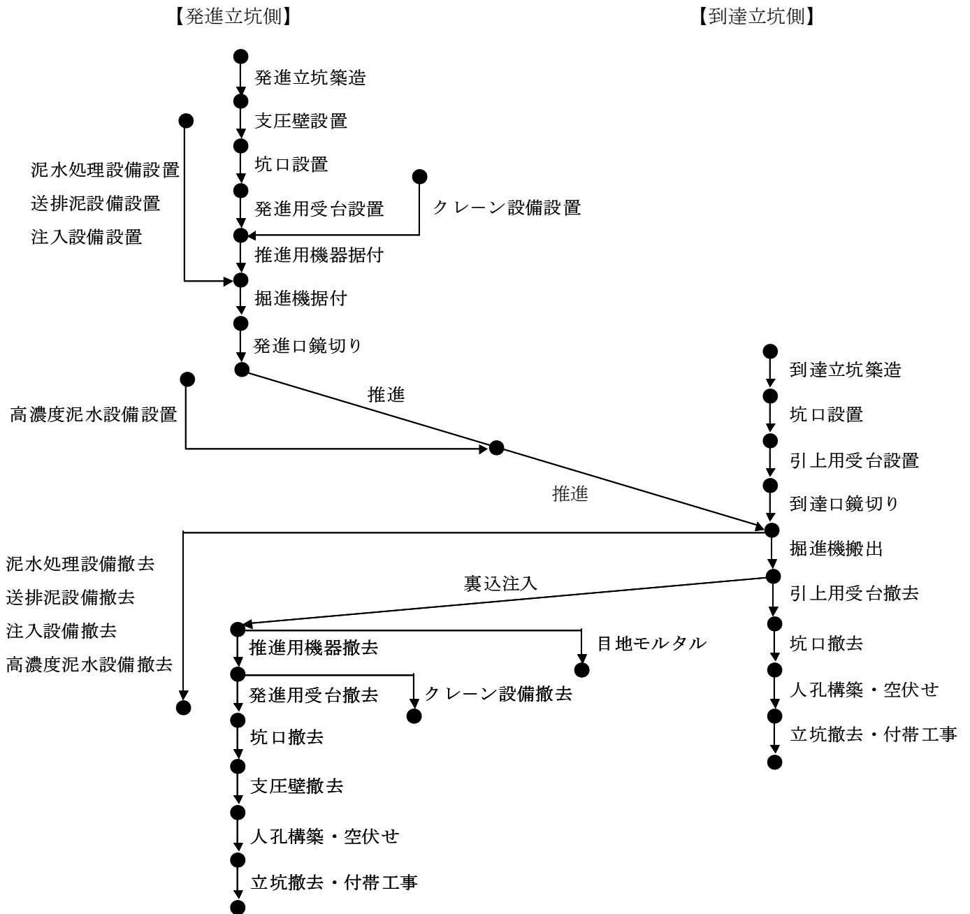
図 1 - 2 施工方式切替の場合の施工手順図（例）
