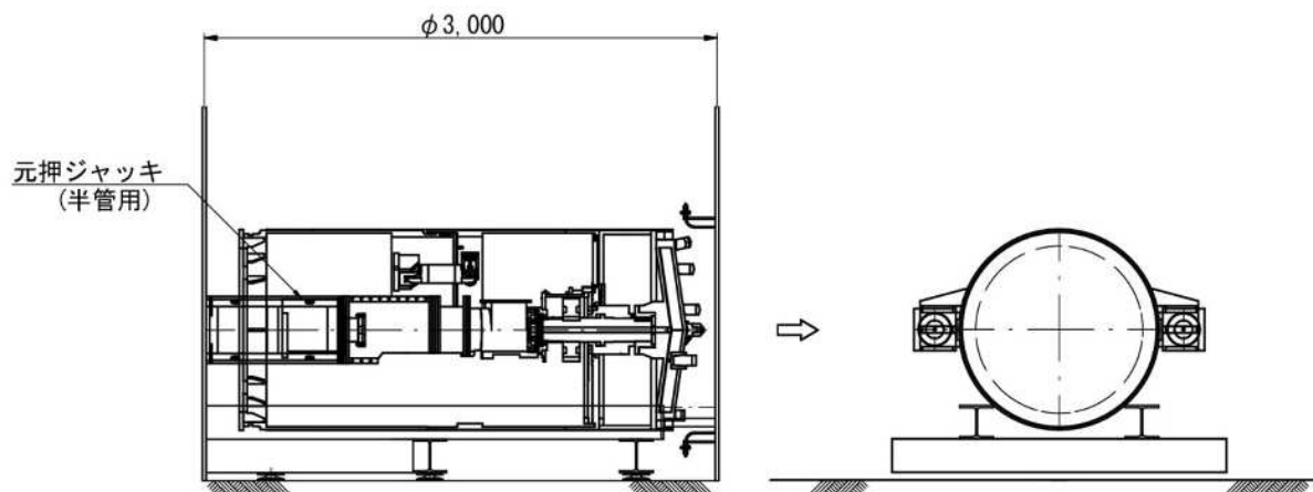
図 9-5 掘進機発進設備
