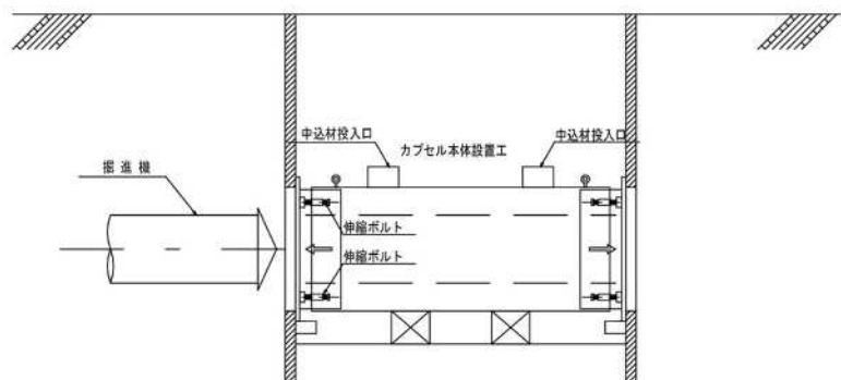
図 9-16 施工手順図－1
