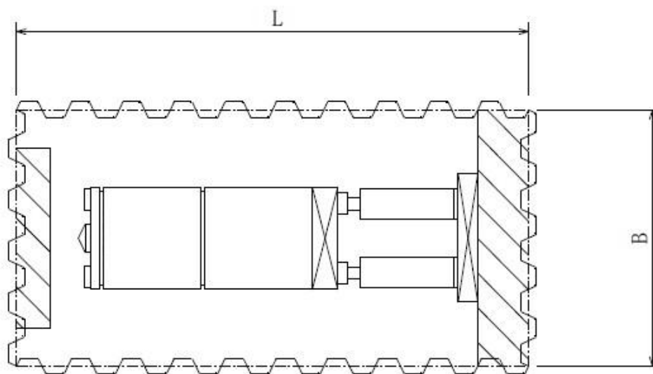
図 7-1 発進・到達立坑(鋼矢板)
