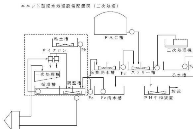
図4-3 ユニット型泥水処理設備配置図(二次処理)
