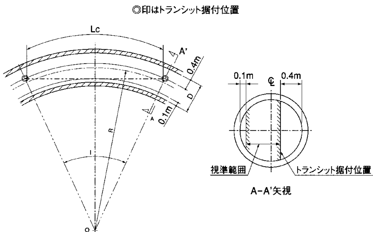
図 6-1 曲線区間での 1 回当たりの測量長・曲線長の関係
