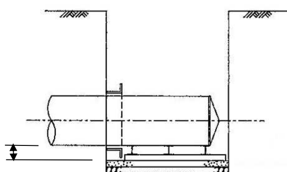
図 7-5 到達立坑
