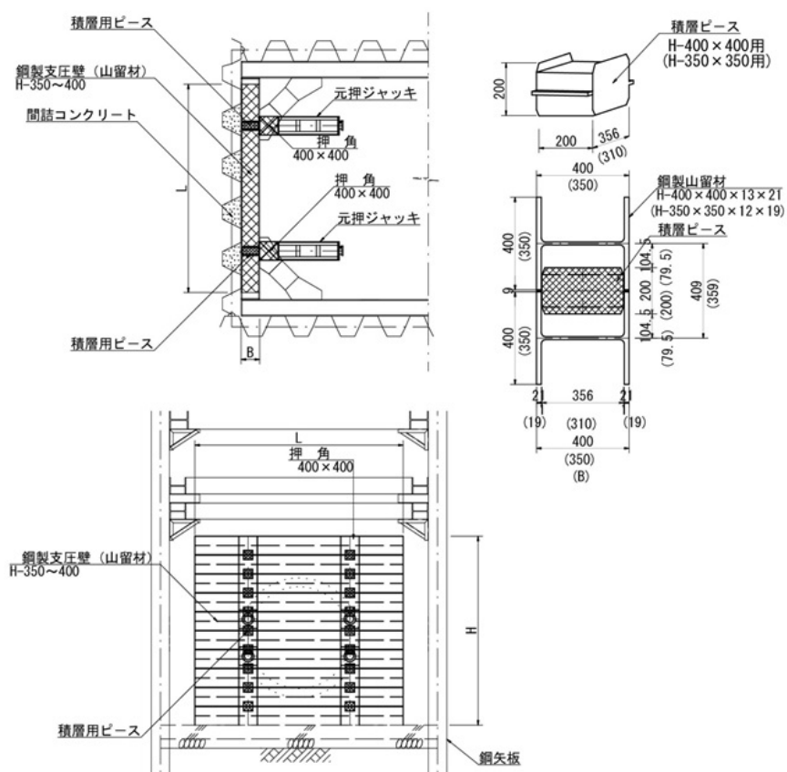
図 9-15 矩形立坑での使用例
