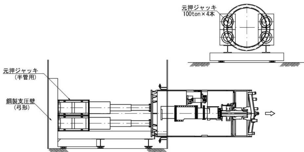
図 9-6 掘進機発進
